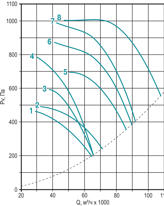
График 60. Аэродинамические характеристики вентилятора /FA.H12.112_А4
