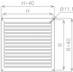
Схема 45. Канальное исполнение
