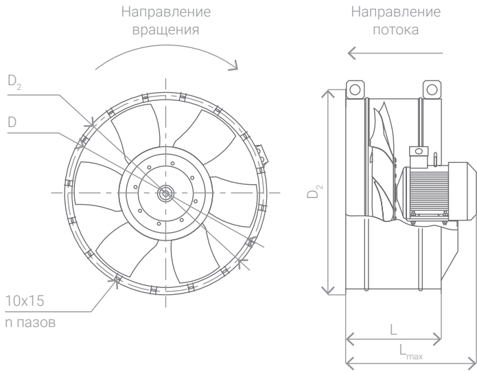
Схема 35. Исполнение AX.F
