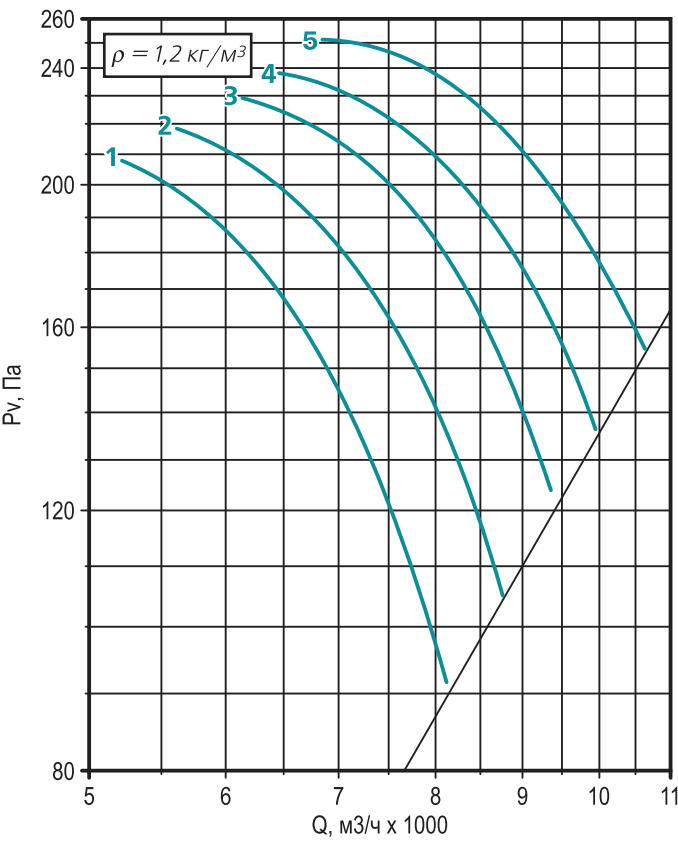
График 39. Аэродинамические характеристики вентилятора /FA.R06.056
