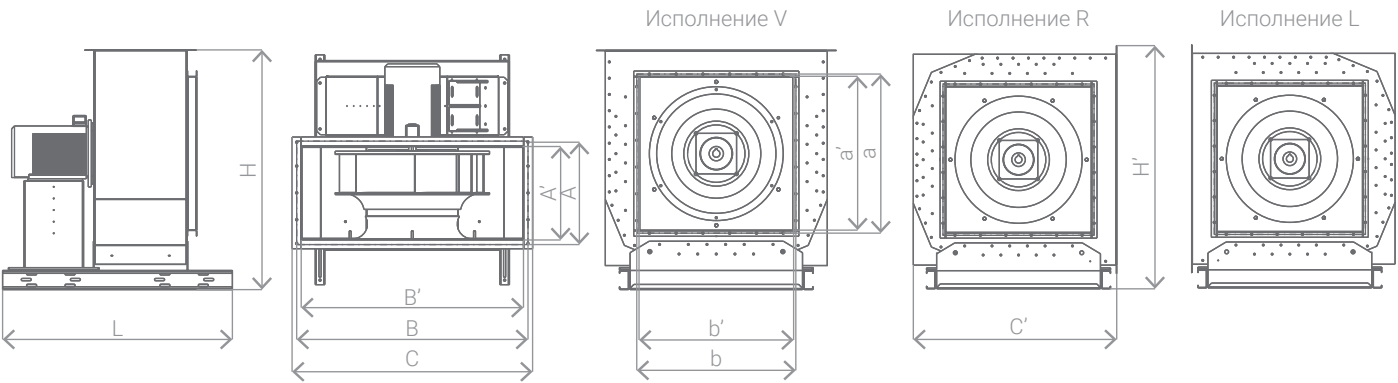
Схема 10. Габаритные и присоединительные характеристики вентиляторов WURFEL SE.400 (600) /FR_
