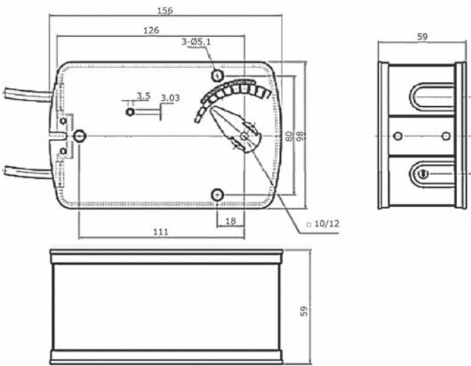
Схема 47. Габаритные размеры электроприводов MB24 / MB220
