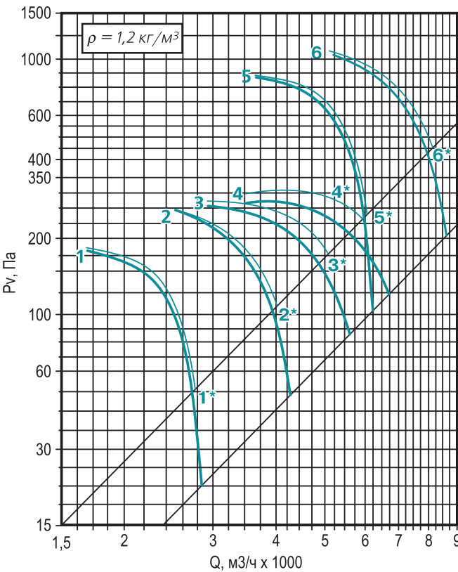
График 28. Аэродинамические характеристики вентилятора /FA.R16.045
