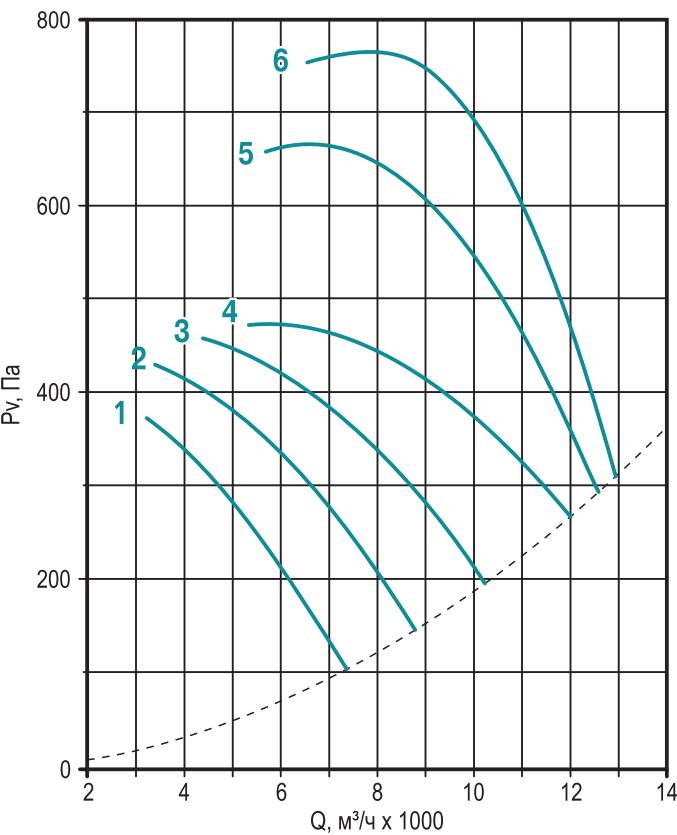
График 48. Аэродинамические характеристики вентилятора /FA.H12.045
