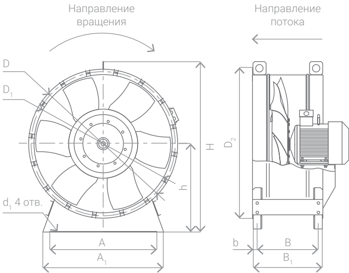
Схема 34. Исполнение AX.S
