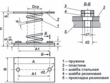
Схема 22. Виброизолятор
