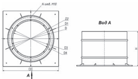
Схема 24. Стакан монтажный круглый под плоскую кровлю
