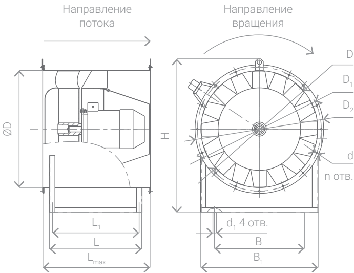
Схема 29. Исполнение AX.S
