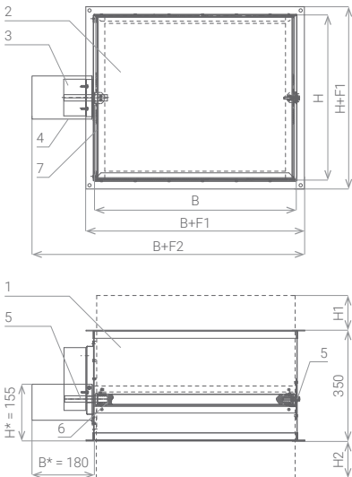
Схема 37. Клапан EI60 (EI90)
