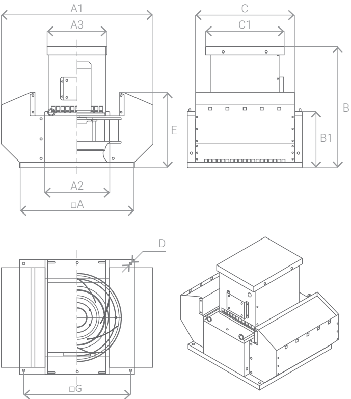
Схема 2. Исполнение с выхлопом вверх SAUGER SE.../FPV
