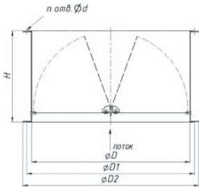
Схема 25. Клапан обратный. Горизонтальное исполнение
