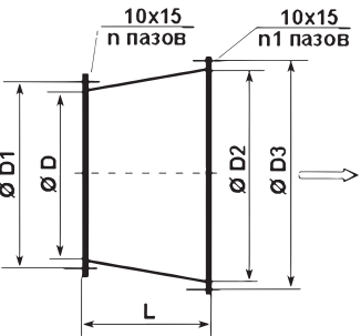
Схема 17. Диффузор на выхлопе
