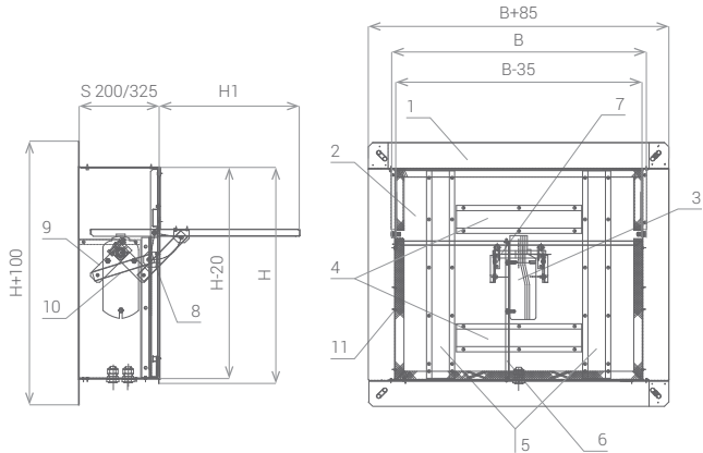
Схема 40. Стеновой клапан E90 (E120, E180)
