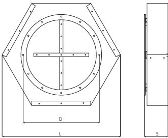
Схема 18. Защитная крыша от осадков
