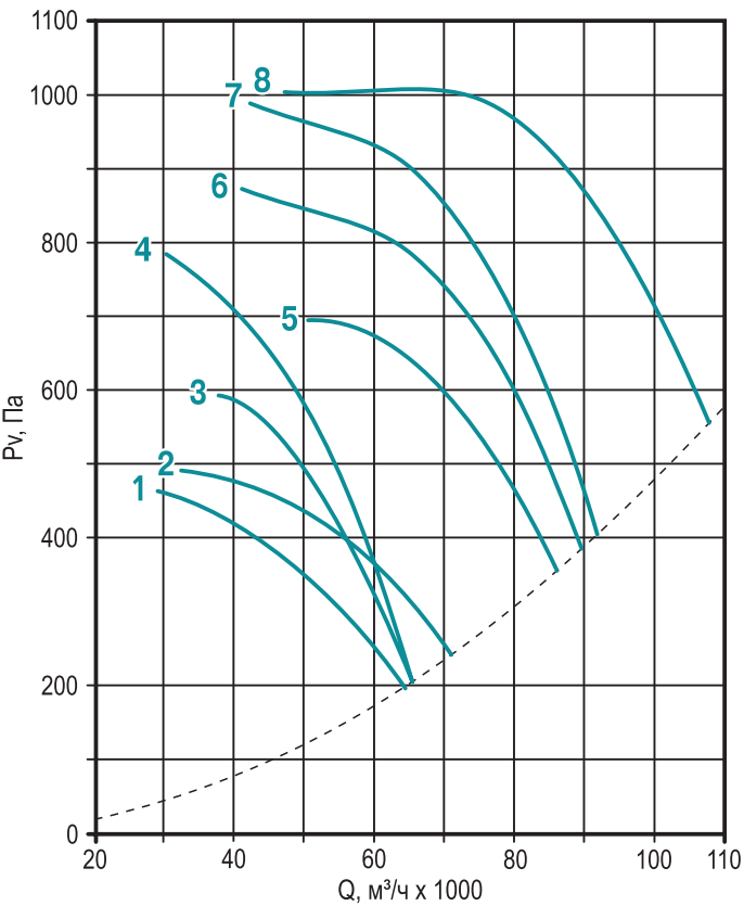
График 60. Аэродинамические характеристики вентилятора /FA.H12.112_А4
