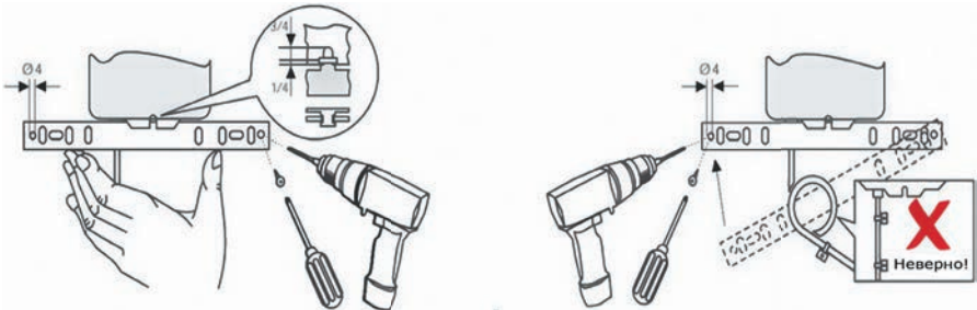
Схема 50. Руководство по монтажу
