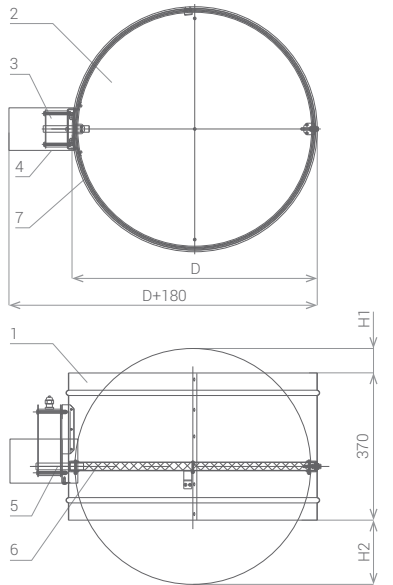
Схема 39. Клапан EI60 (EI90)
