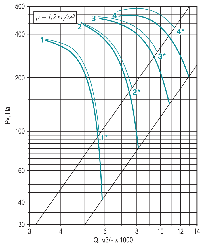
График 30. Аэродинамические характеристики вентилятора /FA.R16.056
