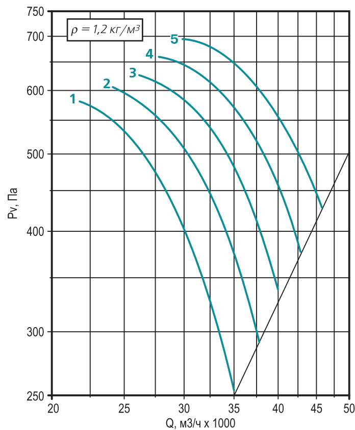
График 43. Аэродинамические характеристики вентилятора /FA.R06.090
