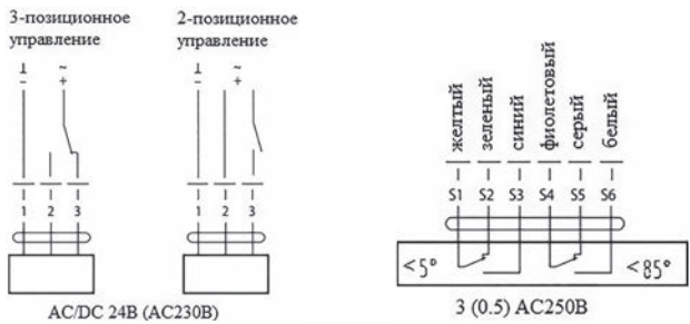
Схема 53. Схема электрических подключений
