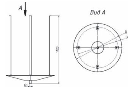
Схема 23. Поддон круглый для сбора конденсата
